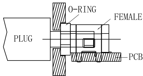
組裝面板防水示意图
