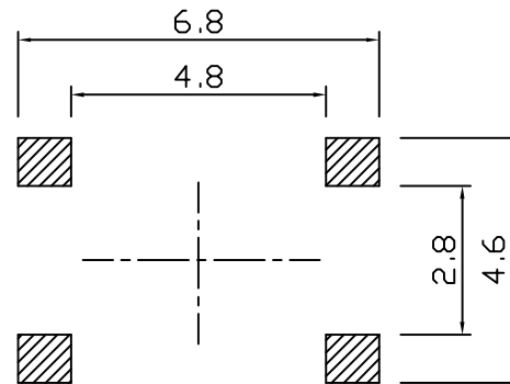
PCB. 焊接图
